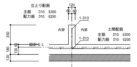
基礎断面詳細図 縮尺 1:30
