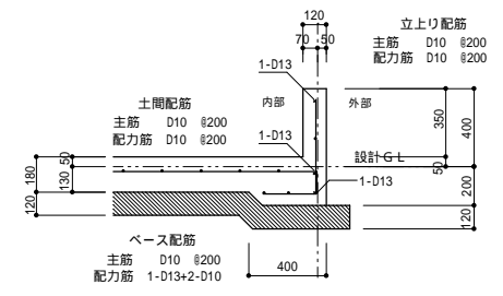
基礎断面詳細図 縮尺 1:30
