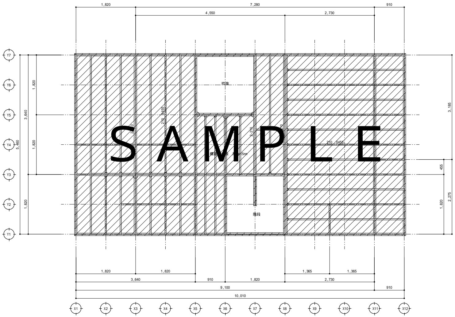
2階床伏図 縮尺 1:50
